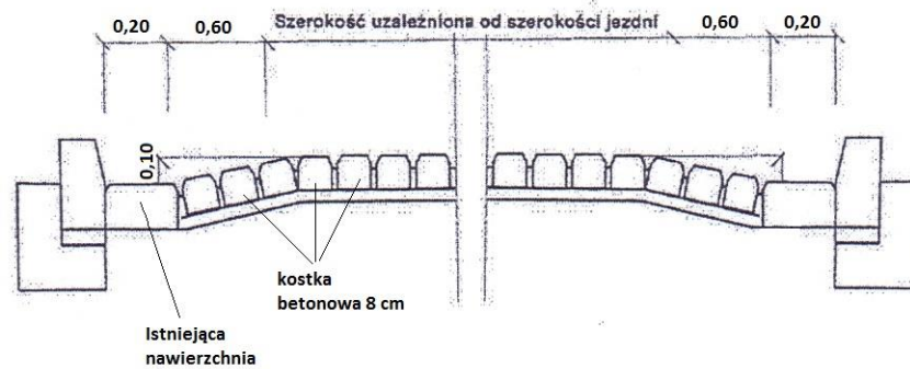
Przekrój poprzeczny B - B
